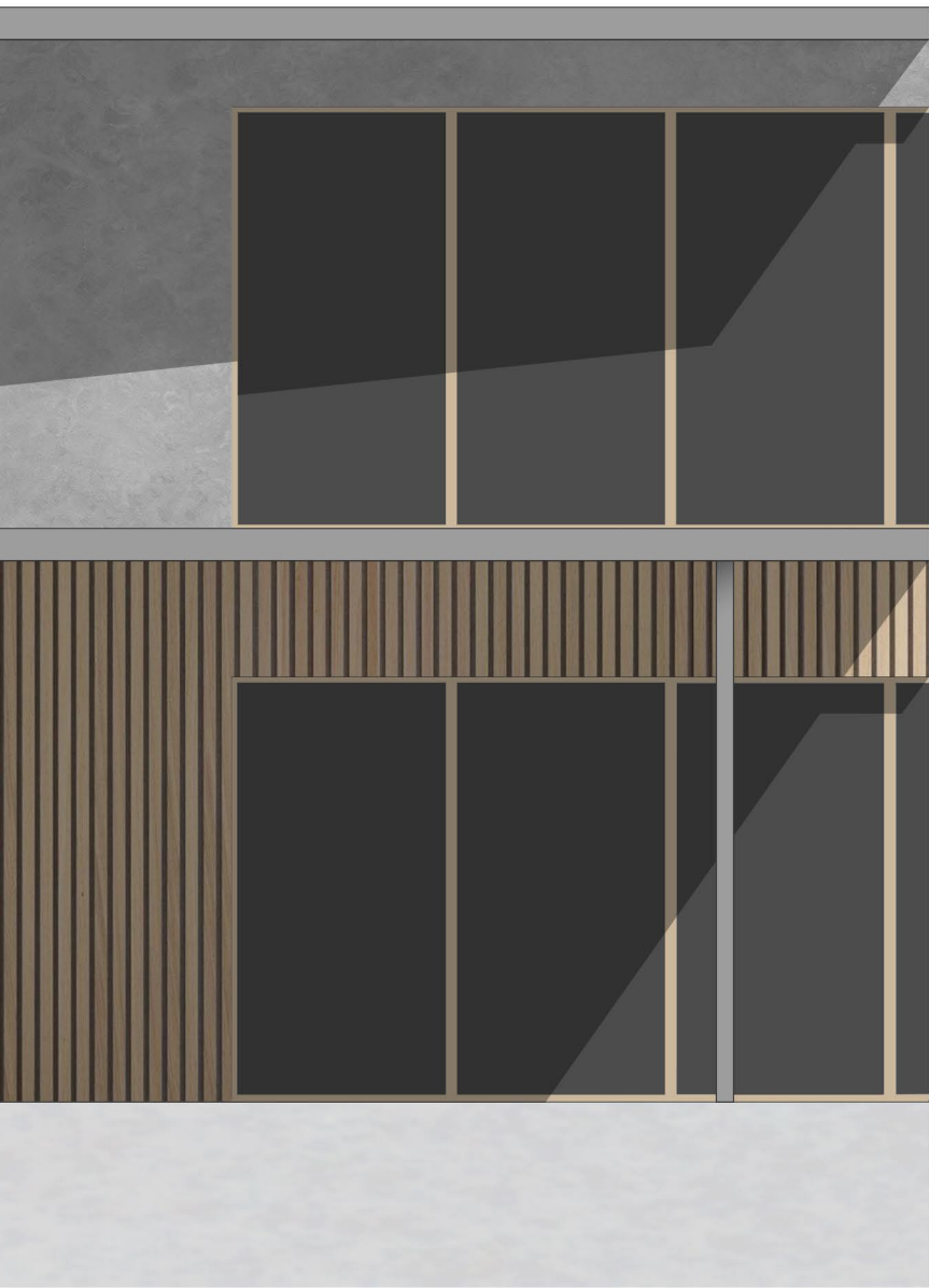
homlokzat részlet M=1:50
