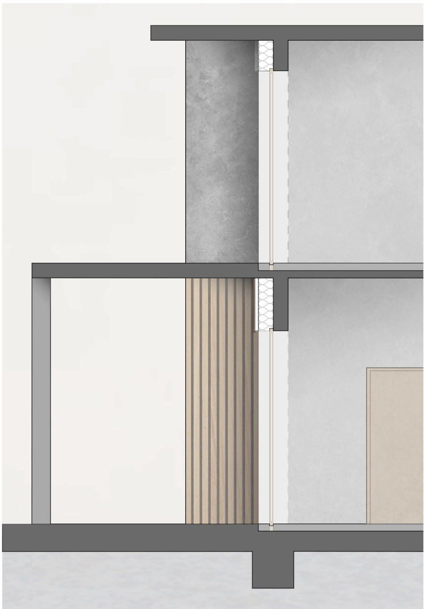
c-c metszet M=1:50
