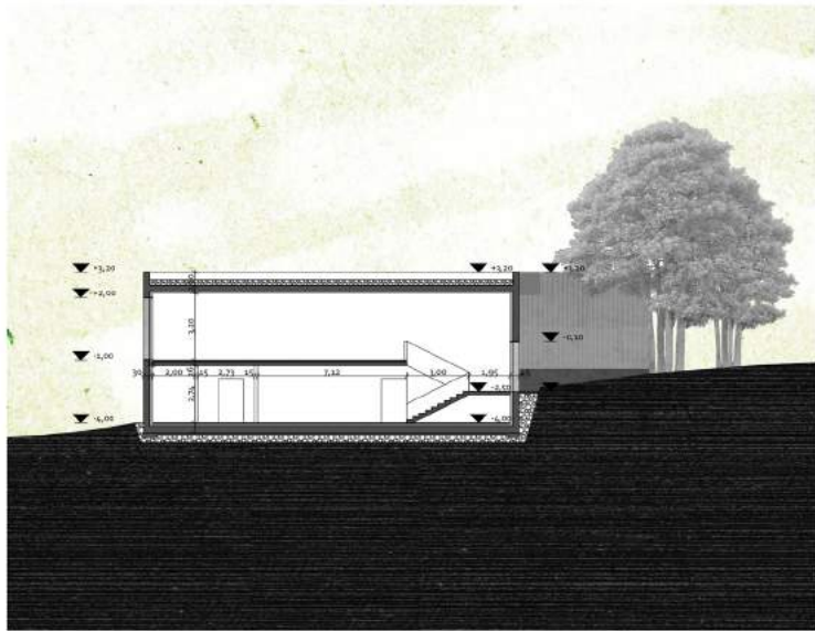
Amerigo Tot Telep. alkotótér 10-10 metszete m=1:100
