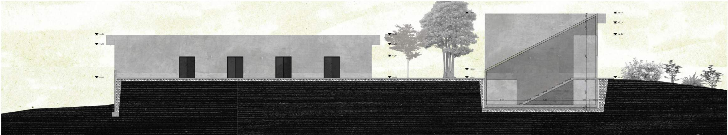
Amerigo Tot Művésztelep. kávézó és emléképület 1-1 hosszszelvénye 1:100
