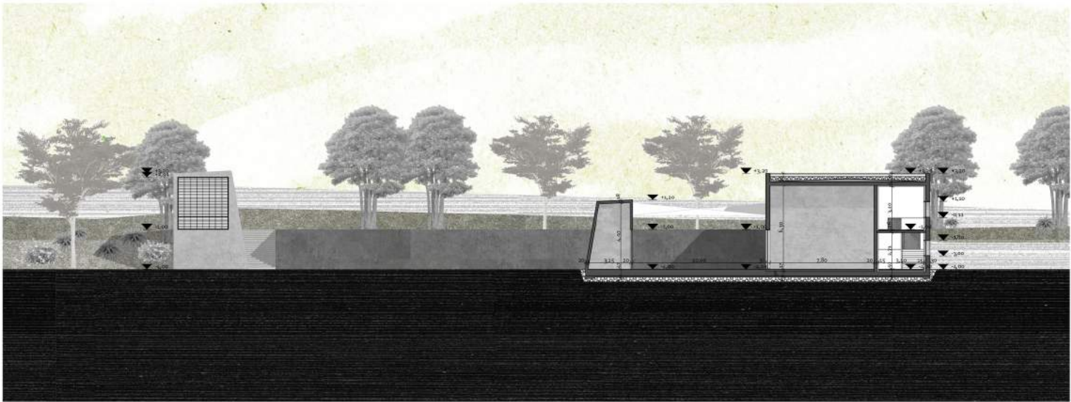
Amerigo Tot Telep. kerámiázó - raktár és alkotótér 5-5 metszete m=1:100
