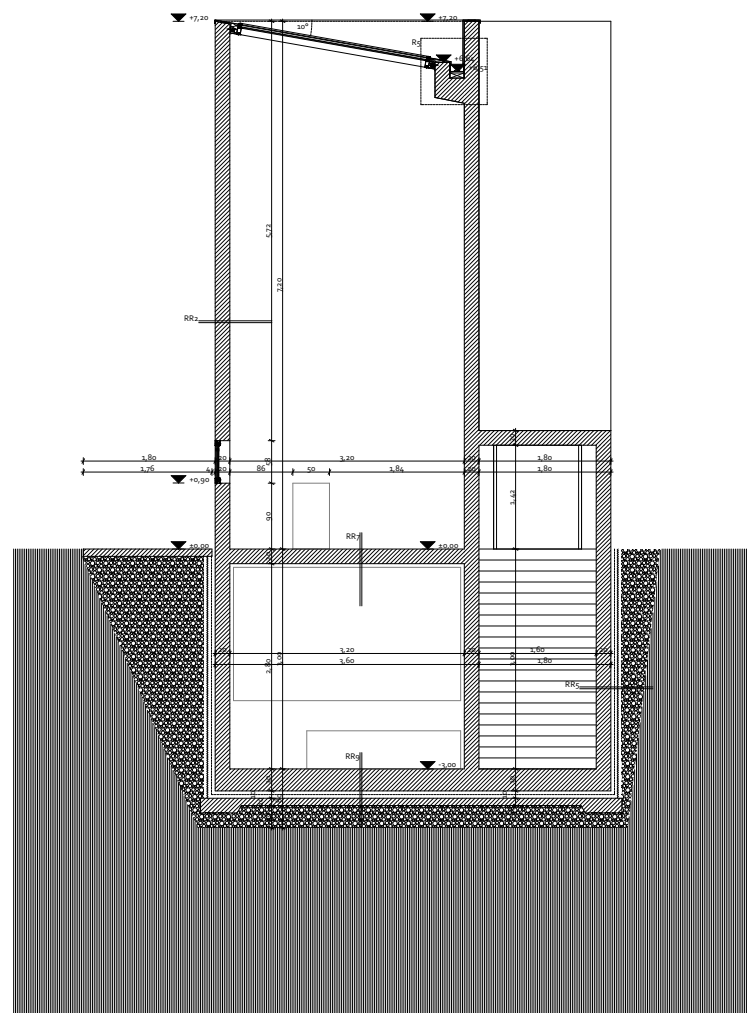
Amerigo Tot Művésztelep. 2-2 emléképület keresztmetszet 1:50
