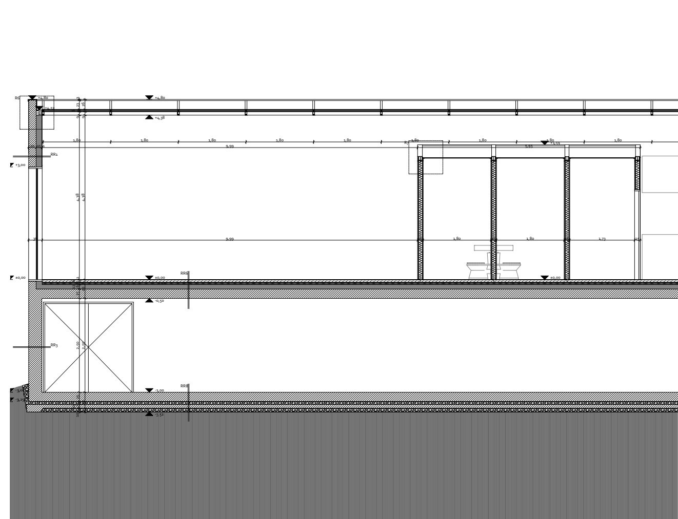
Amerigo Tot Művésztelep. 4-4 kávézó hosszmetset 1:50
