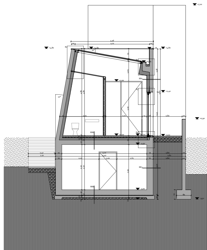
Amerigo Tot Művésztelep. 3-3 kávézó keresztmetszet 1:50
