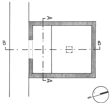
GAJDÁCS PÁL LÁSZLÓ ÉPÍTÉSZE SZABADSÁG ALAPRAJZA, METSZETEI M=1:50
