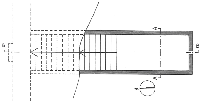
GAJDÁCS PÁL LÁSZLÓ ÉPÍTÉSZE ALAPRAJZ, METSZETEI M=1:50
