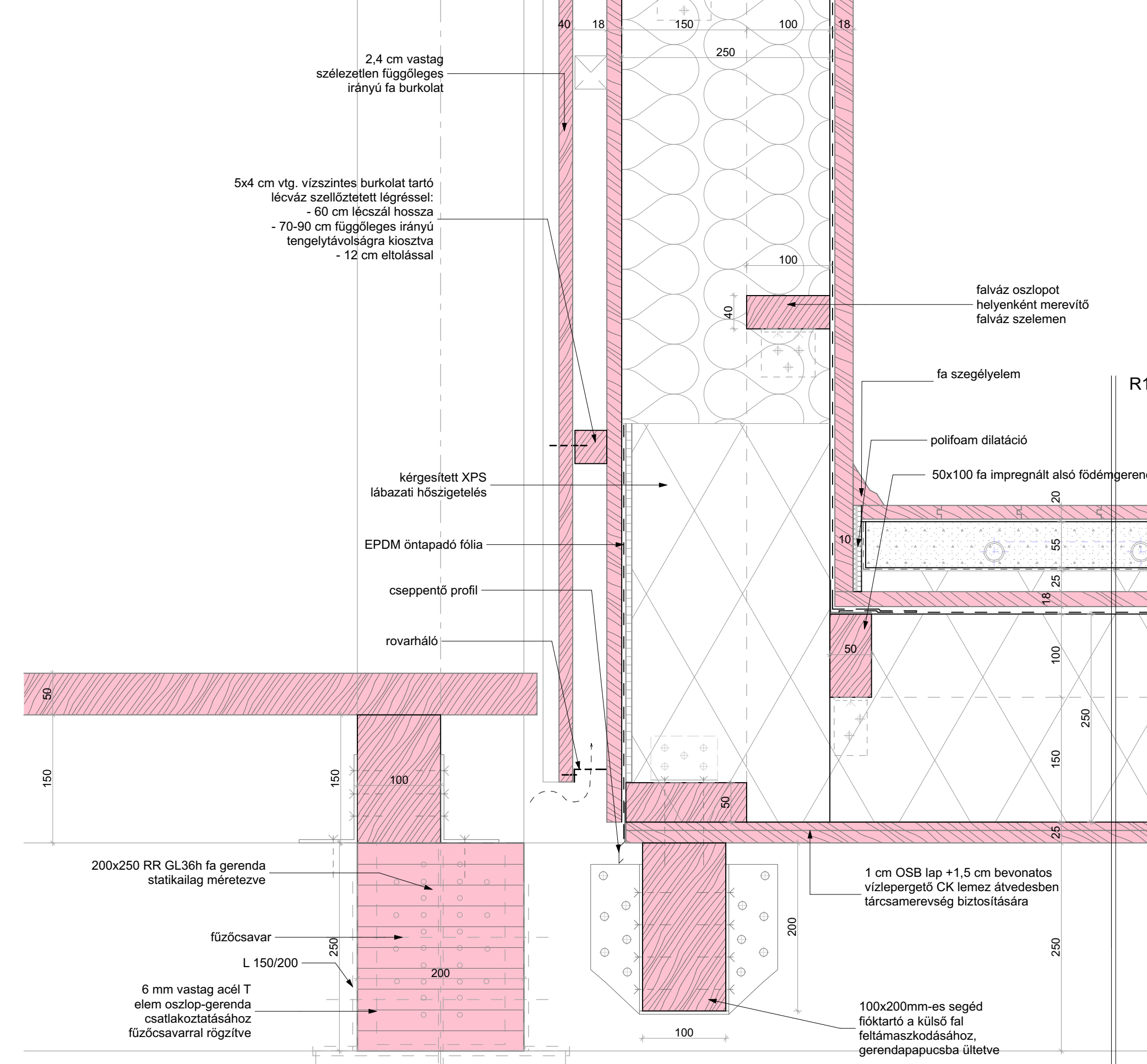
CS4 M 1:5
