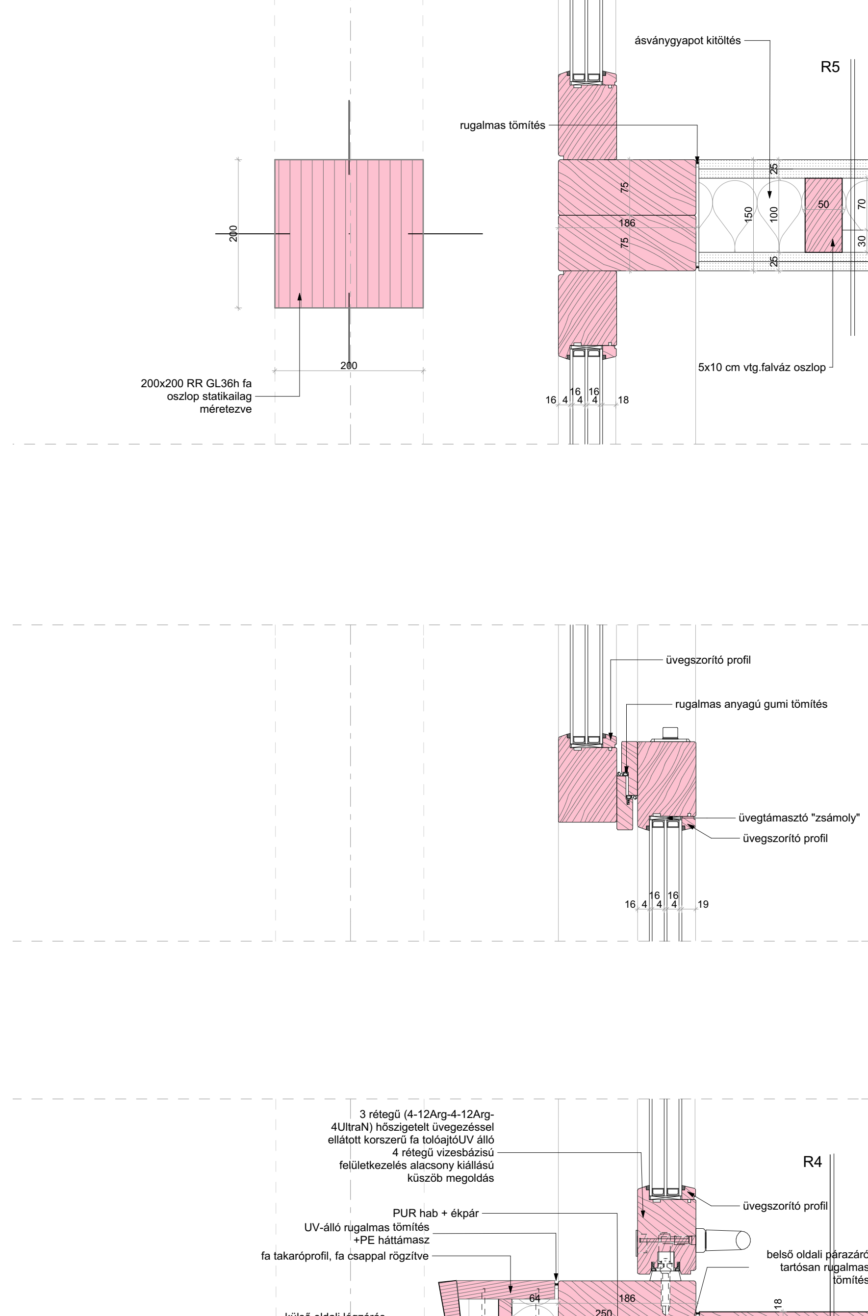
CS7 - CS8_M 1:5
