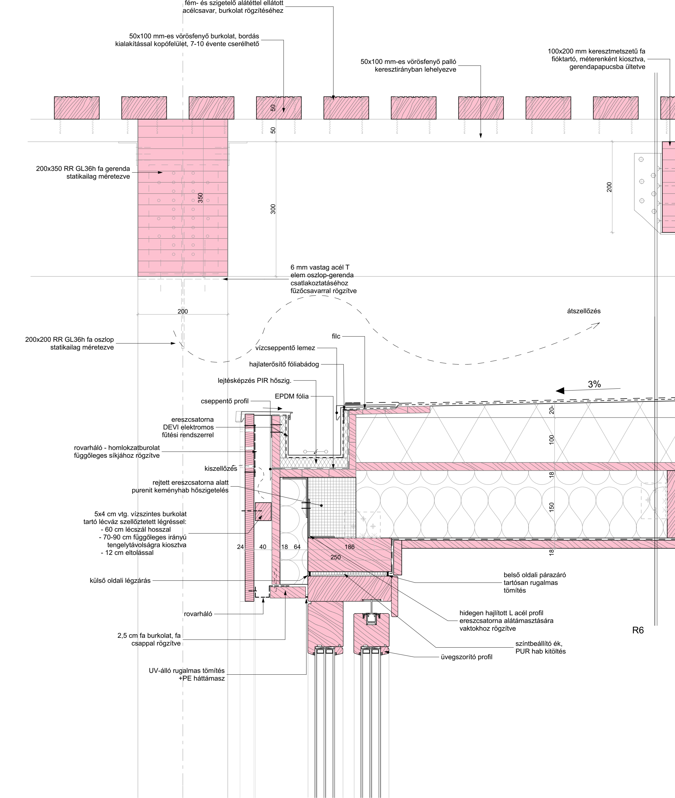
CS2_M 1:5
