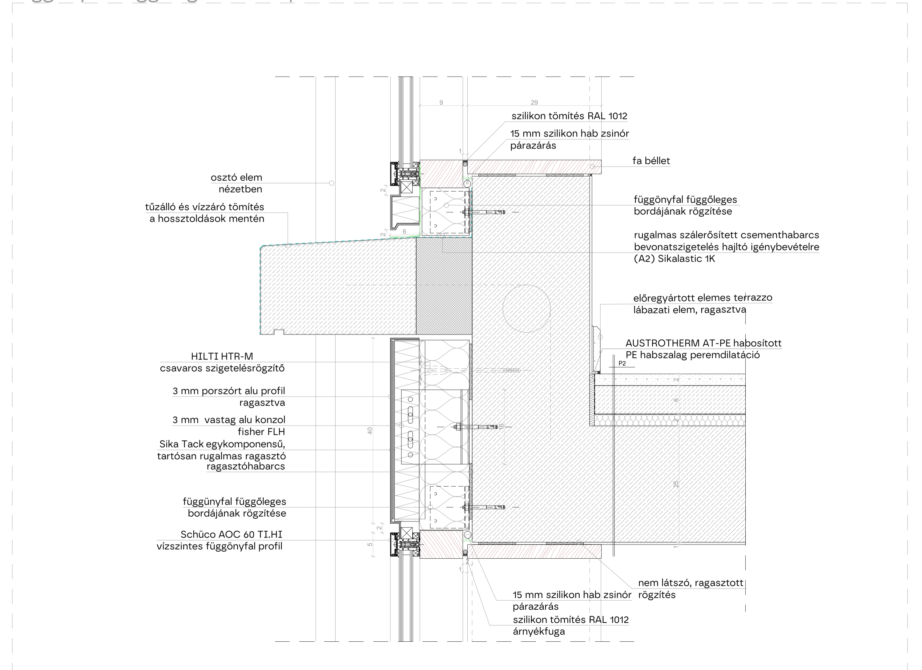
függönyfal függőleges csomópont
