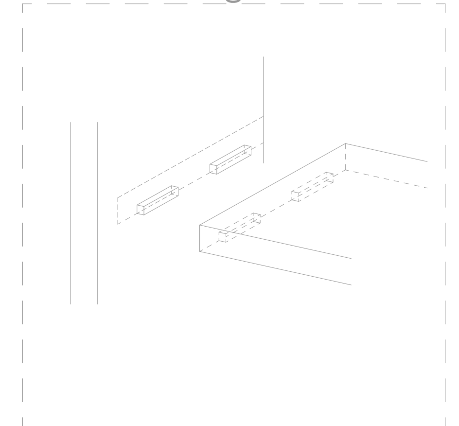
nem látszó rögzítések
