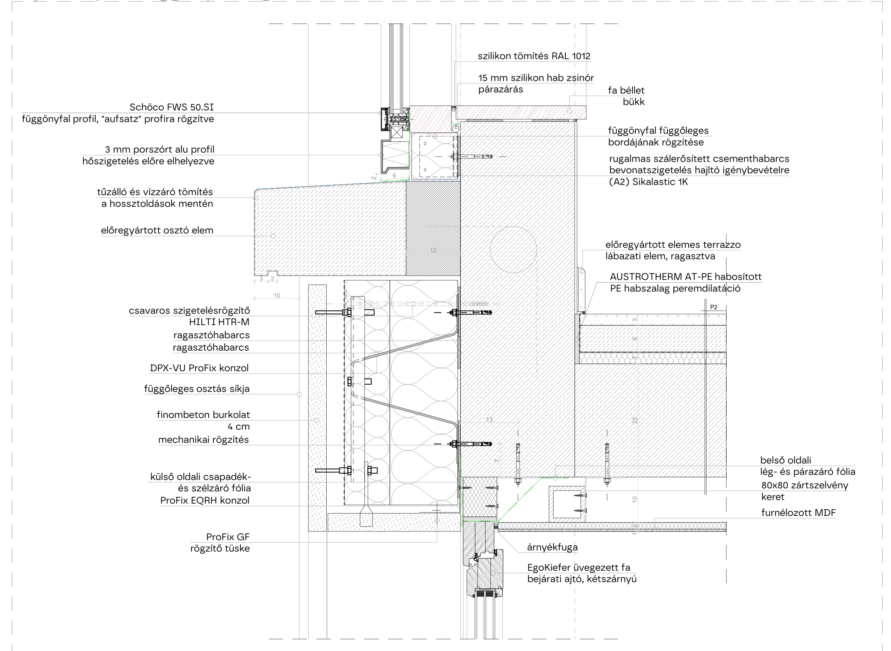
bejárati ajtó - függönyfal rögzítése
