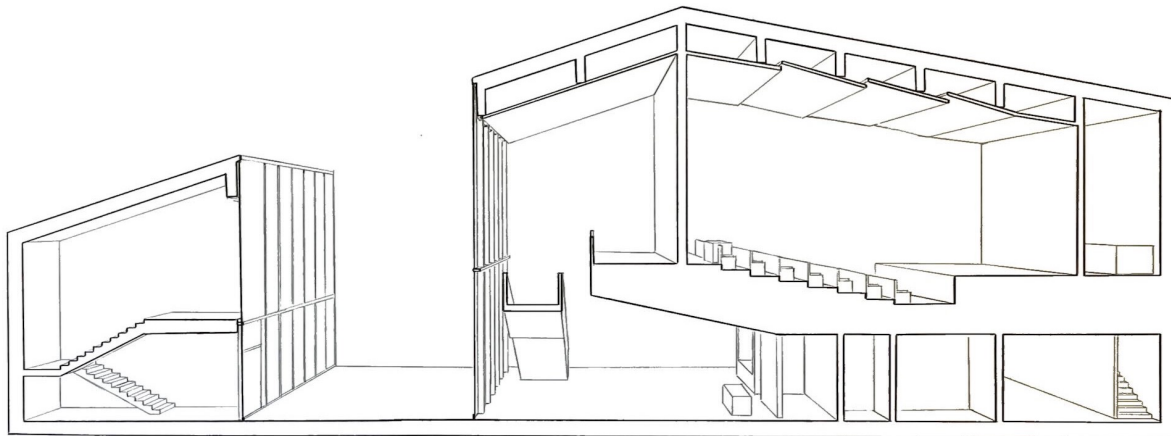
A-A metszet
