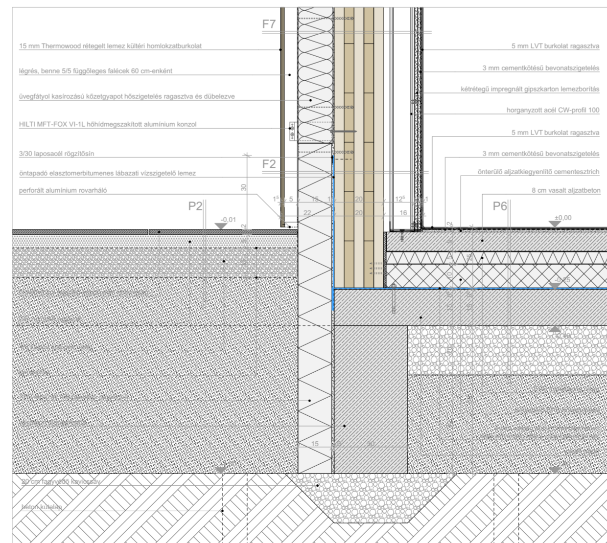
lábázati csomópont a fedett nyitott tér felől
