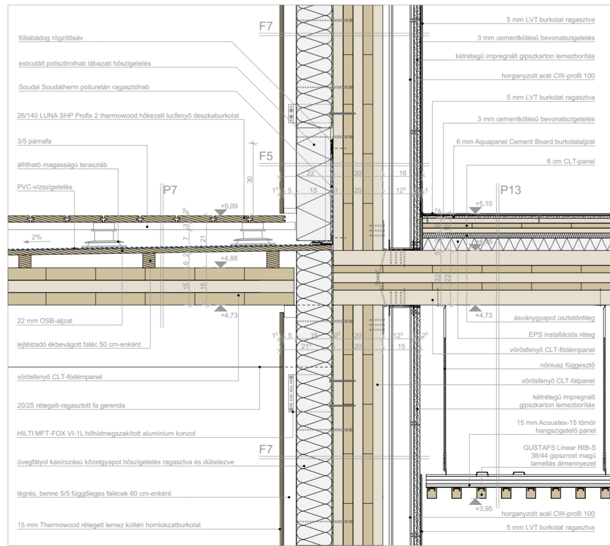
emeleti terasz lábazati csomópont M=1:5
