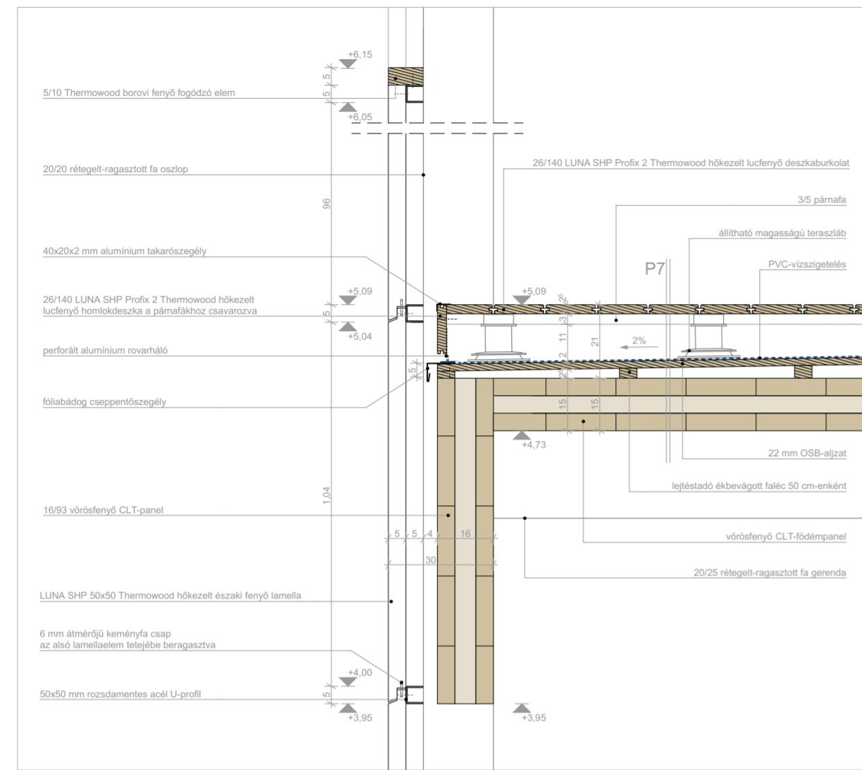
teraszszegély csomópont
