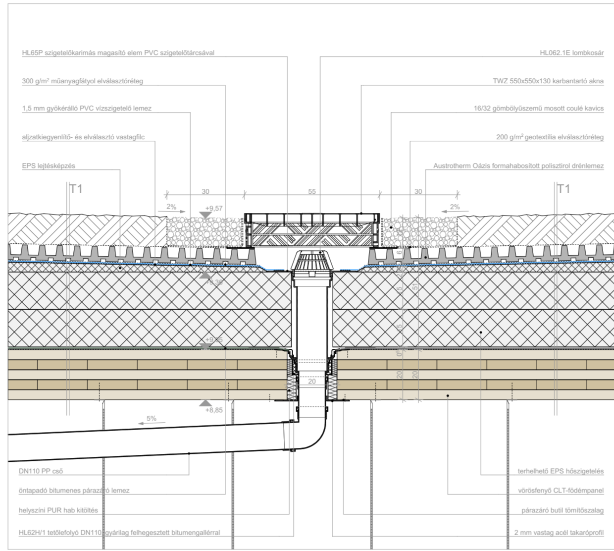
tetőleflyő csomópont M=1:5
