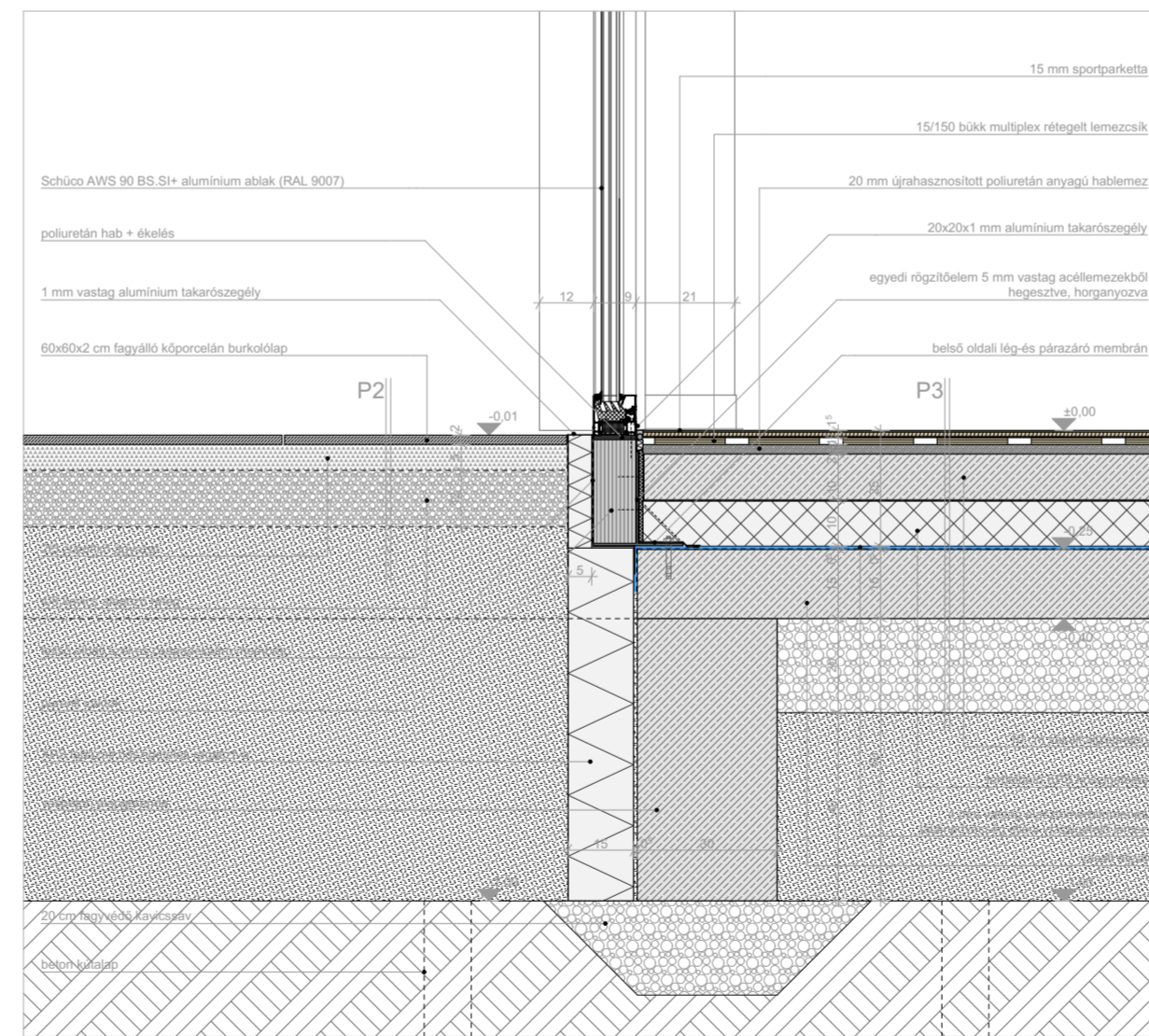
ablak alsó csomópont a fedett-nyitott tér felől
