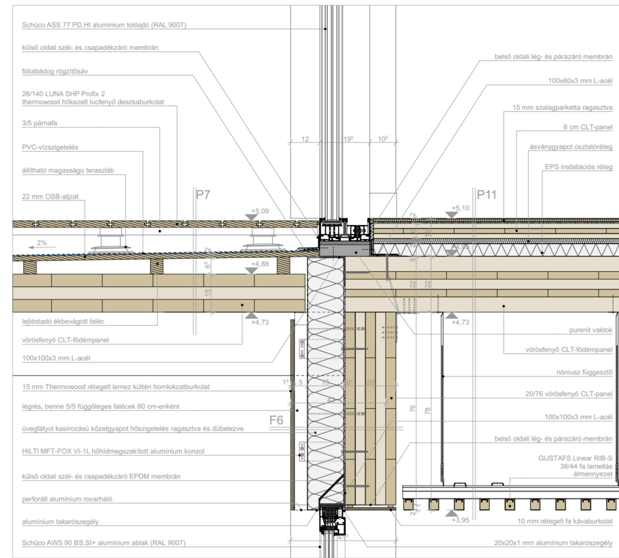
teraszajtó alsó csomópont
