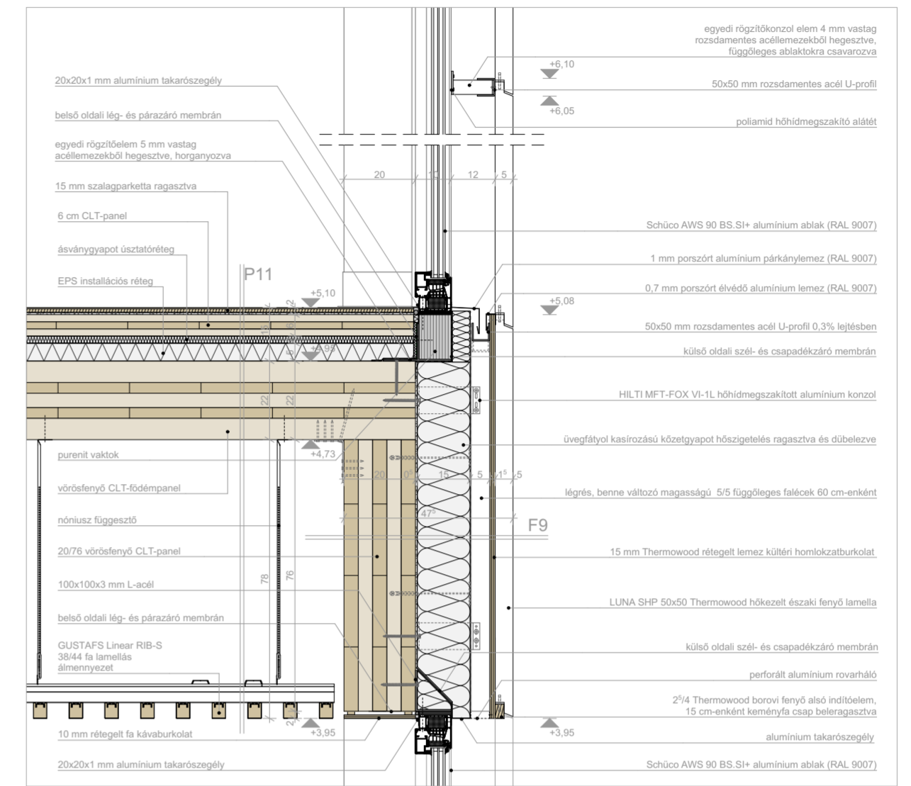
kávészó ablak alsó csomópont
