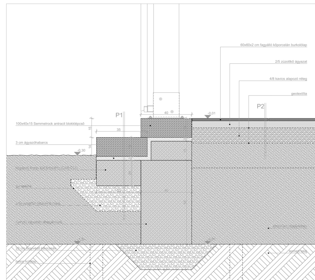
teraszlépcső csomópont
