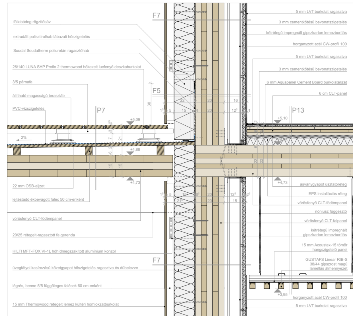
emeleti terasz lábázati csomópont
