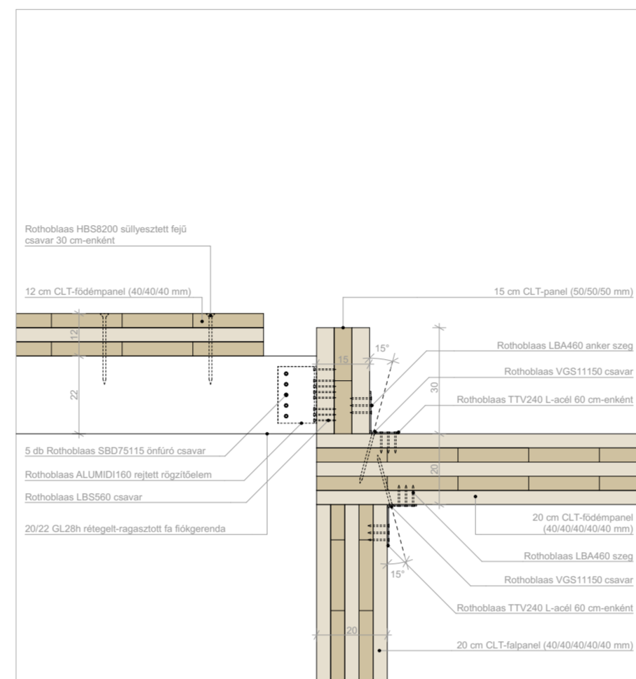
Terasztető és zárófödém szerkezetének kapcsolatai
