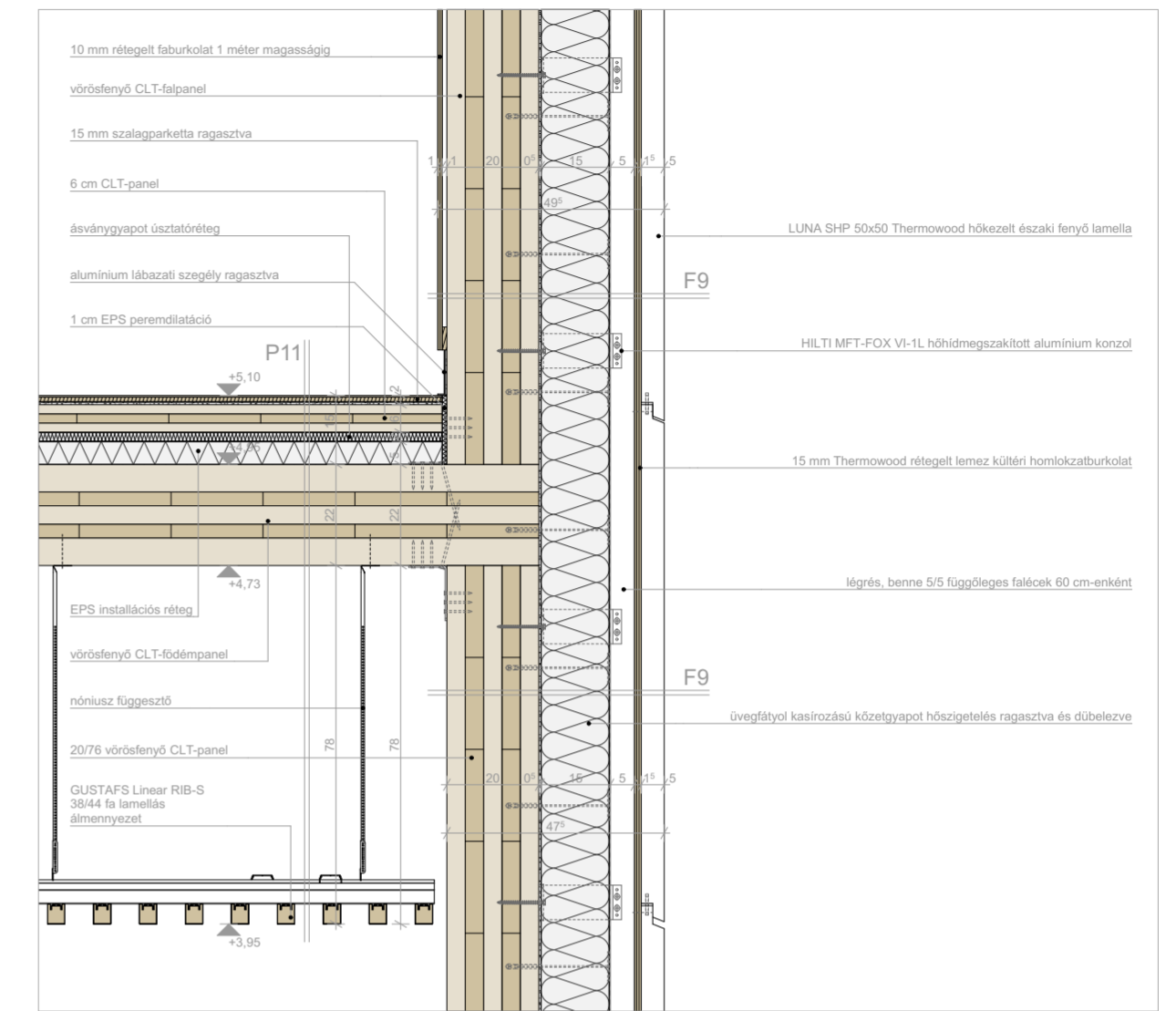
emeletközi földm-fal csomópont
