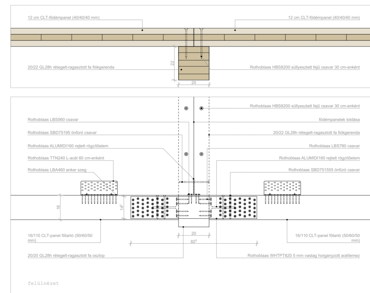
Födémpanelek toldása fókgerendán
