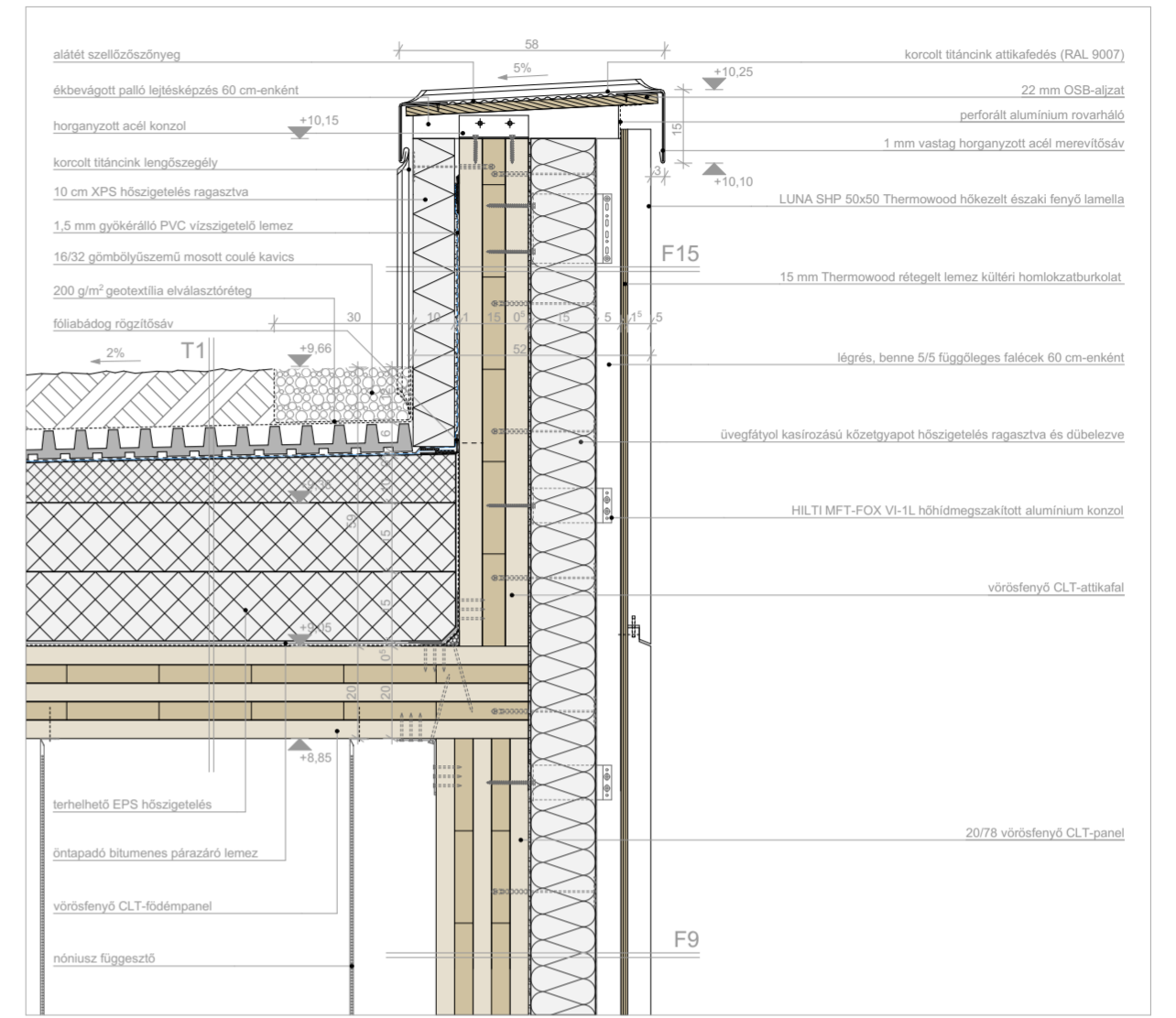
hőszigetelt attika csomópont M=1:5
