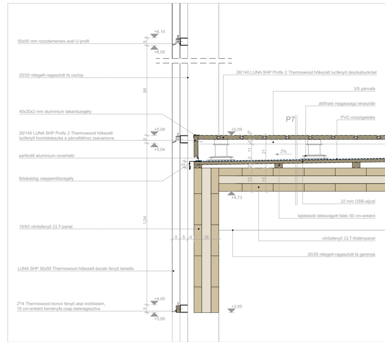
teraszszegély csomópont
