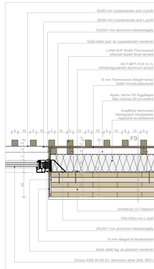
kávézó ablak vízszintes csomópont
