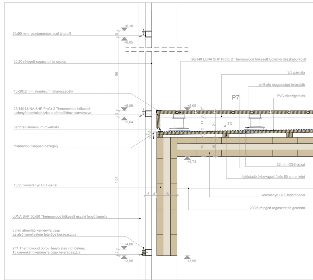
teraszszegély csomópont M=1:5
