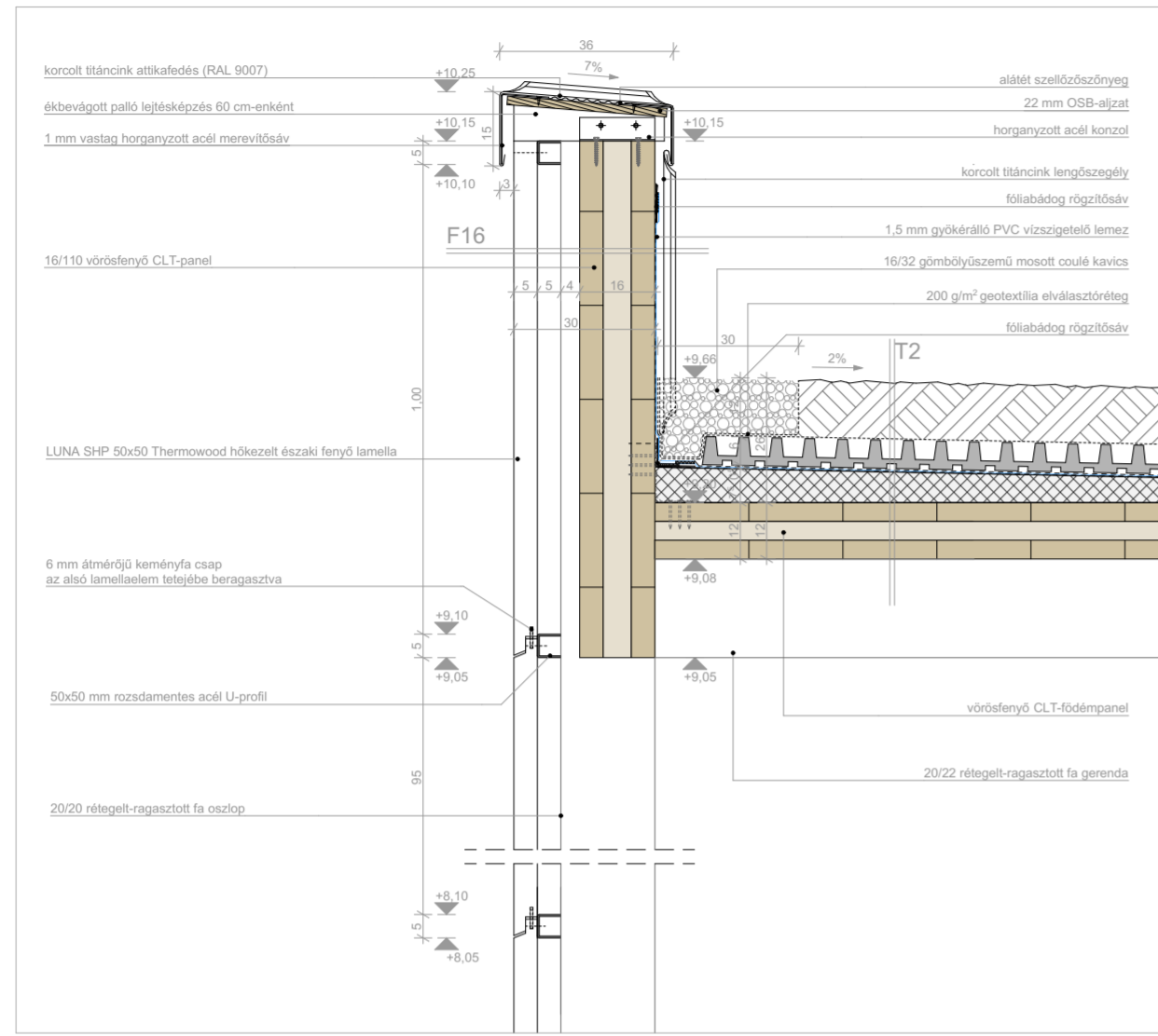
hőszigetetlen attika csomópont M=1:5
