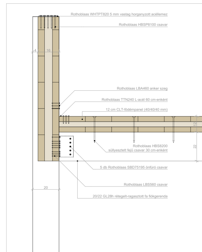
Főtartó-fiókgerenda-födém kapcsolat
