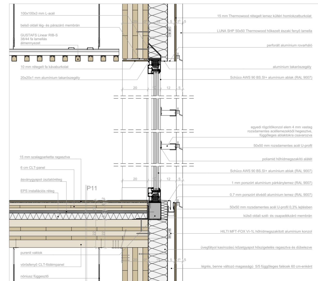
kávézó ablak függőleges csomópontok
