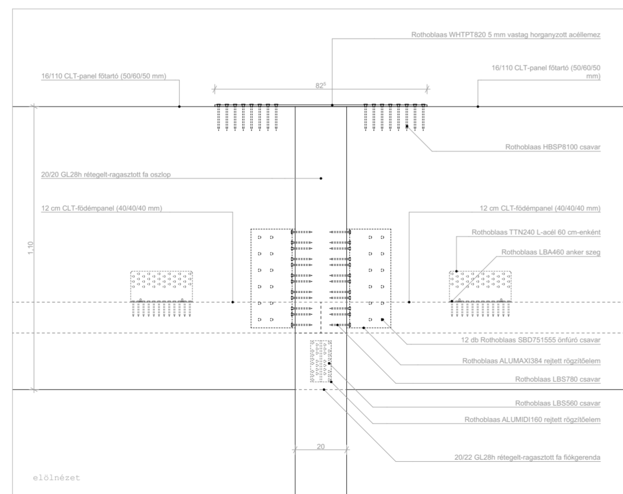
Oszlop-főtartó-fiókgerenda-födém kapcsolat
