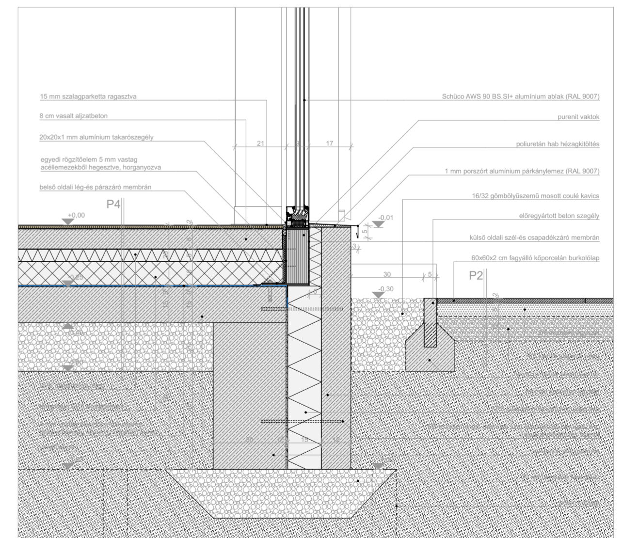
ablak alsó csomópont a sziklafal felől
