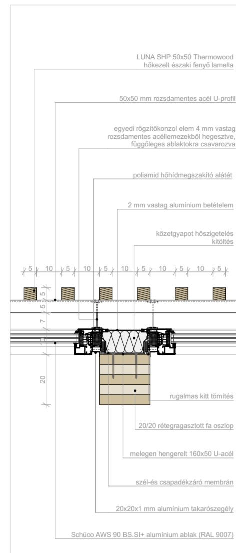
kávézó ablaksorolás csomópont
