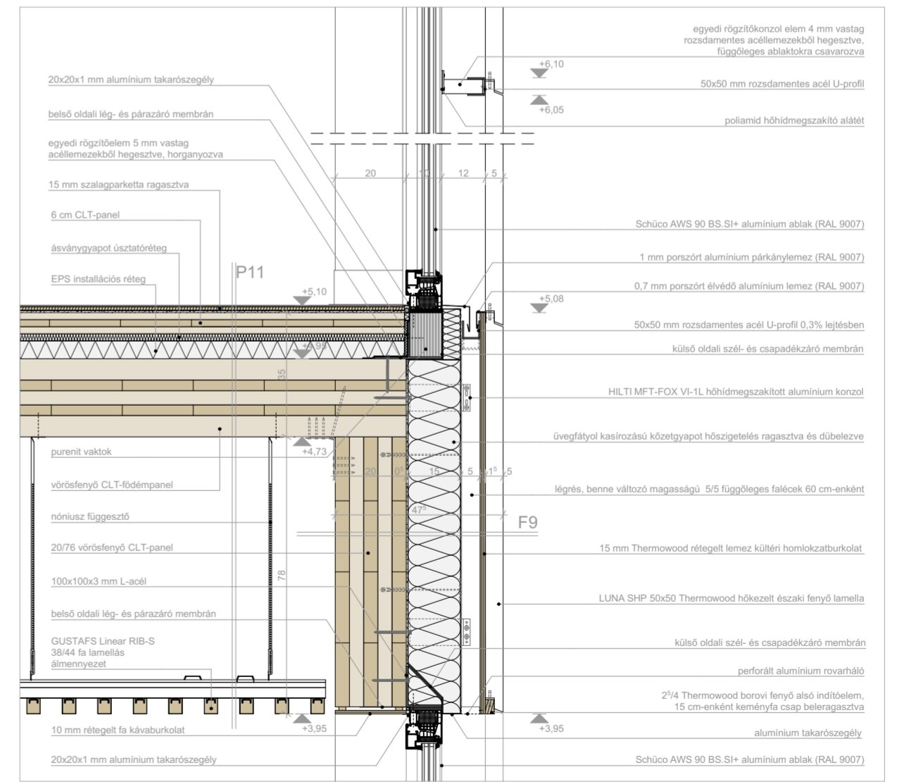
kávészó ablak alsó csomópont M=1:5
