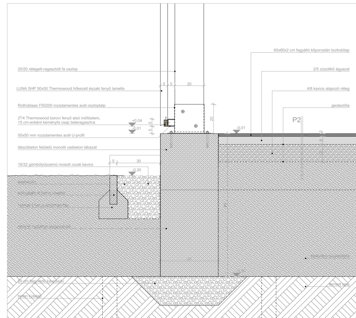
fa oszlop alsó csomópont
