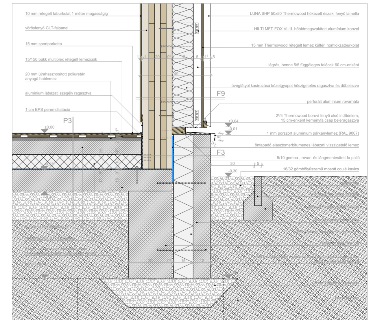
lábazati csomópont a sziklafal felől
