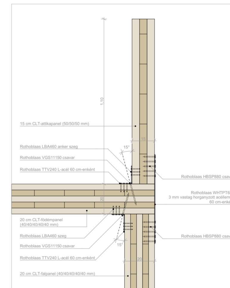
Fal-födém-attika kapcsolat
