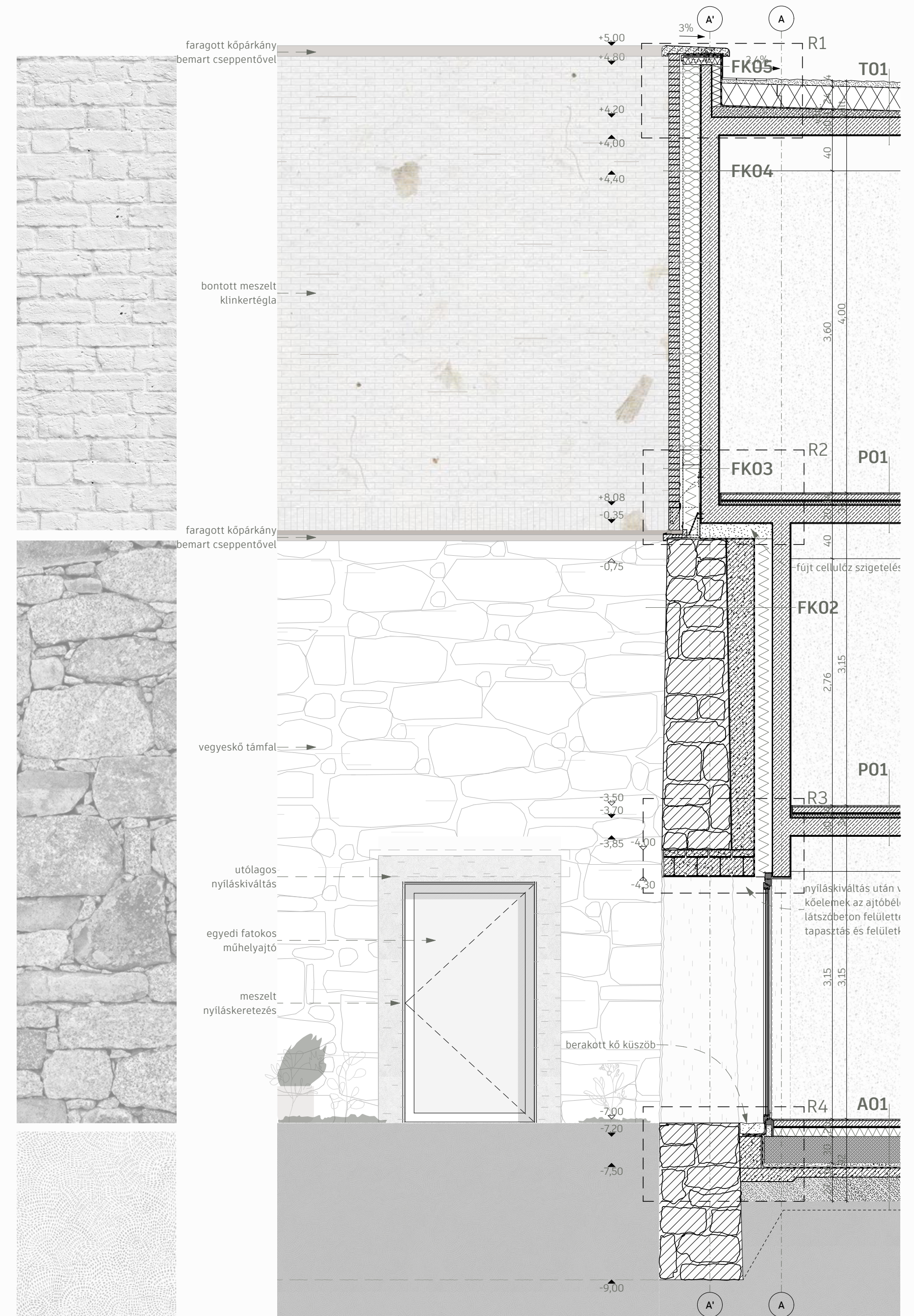
Bábműhely részmet szet és részhomlokzat
