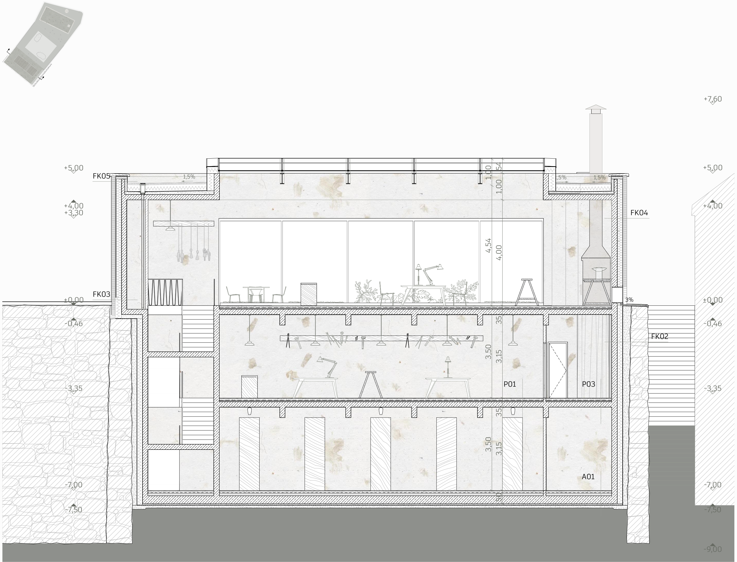
Bábműhely hosszmetset
