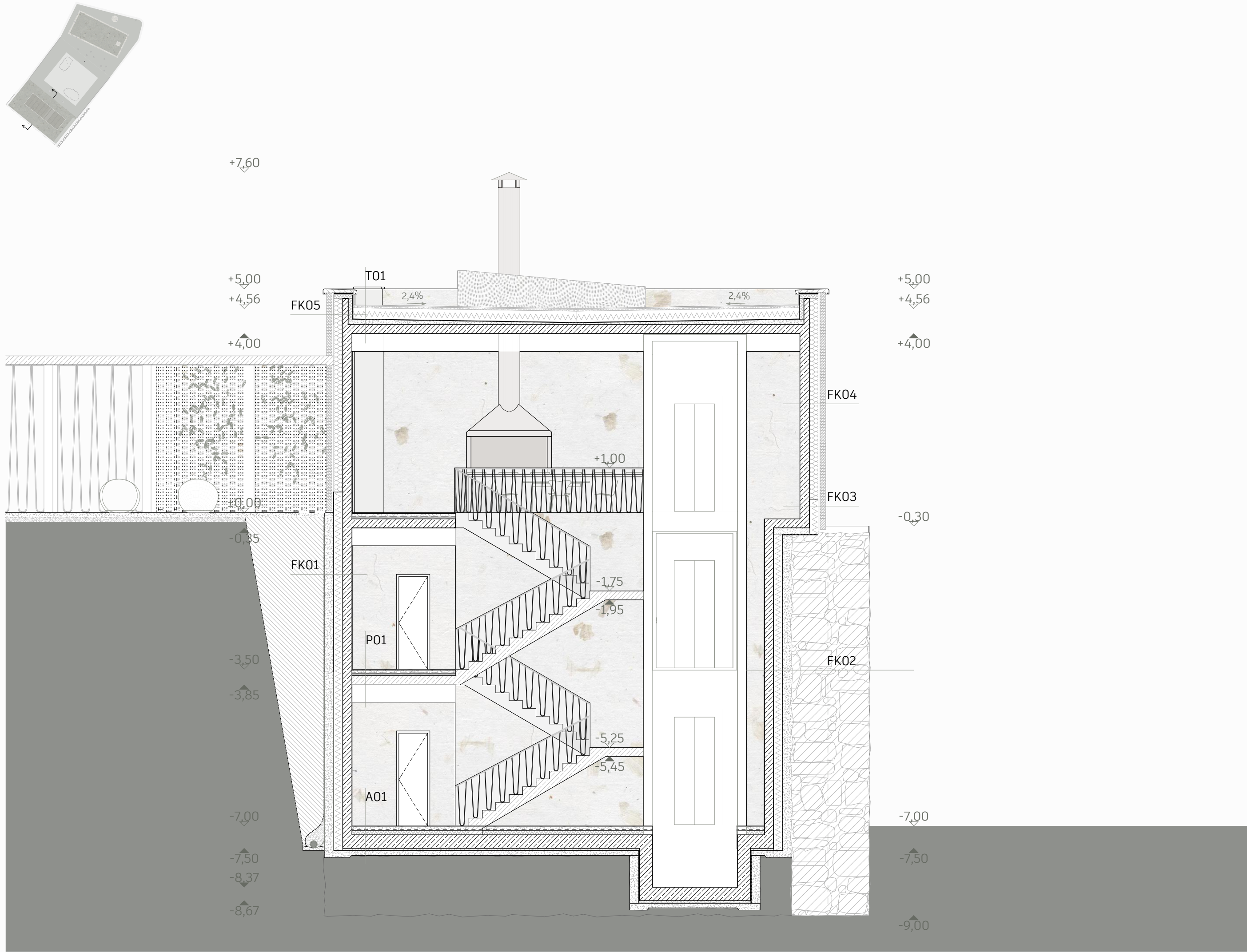
Bábműhely keresztmetszet
