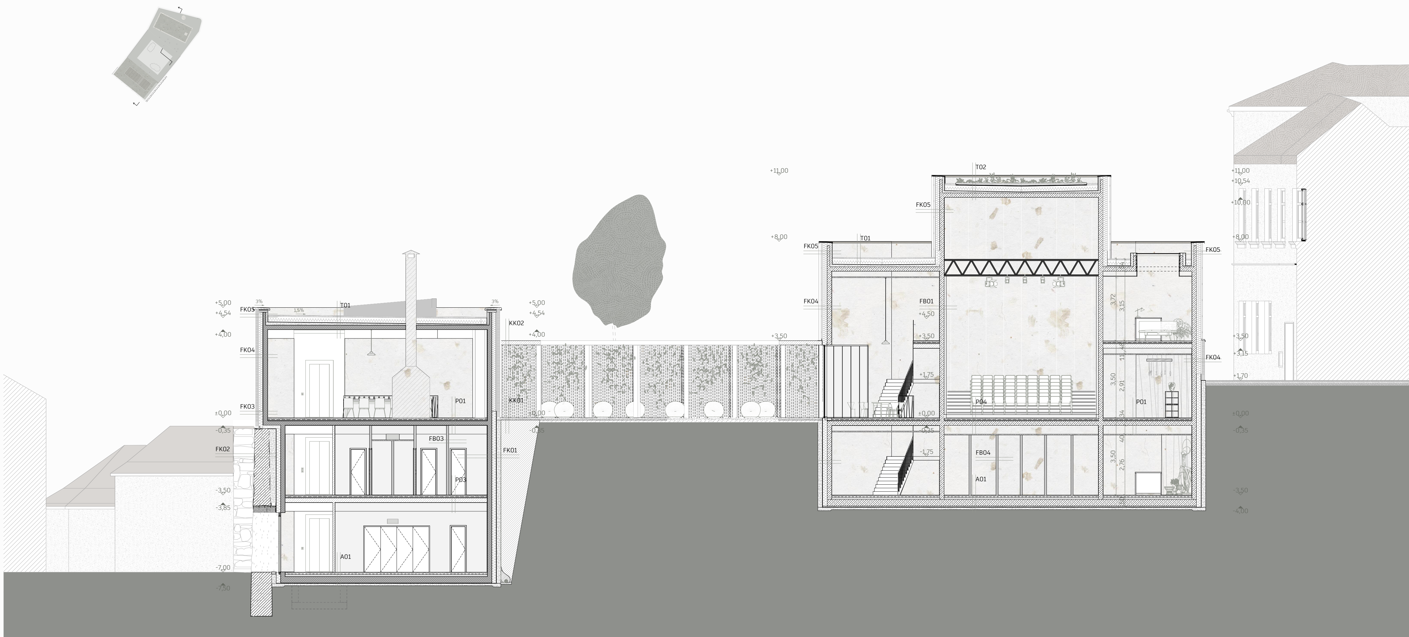
Terepmenti hosszmetset
