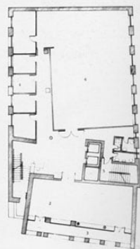
Planta primera / First floor plan
