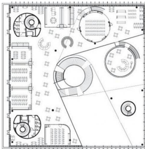
Ørestad Gymnasium, Kopenhagen, Dánia, 3XN Architects, 2007
