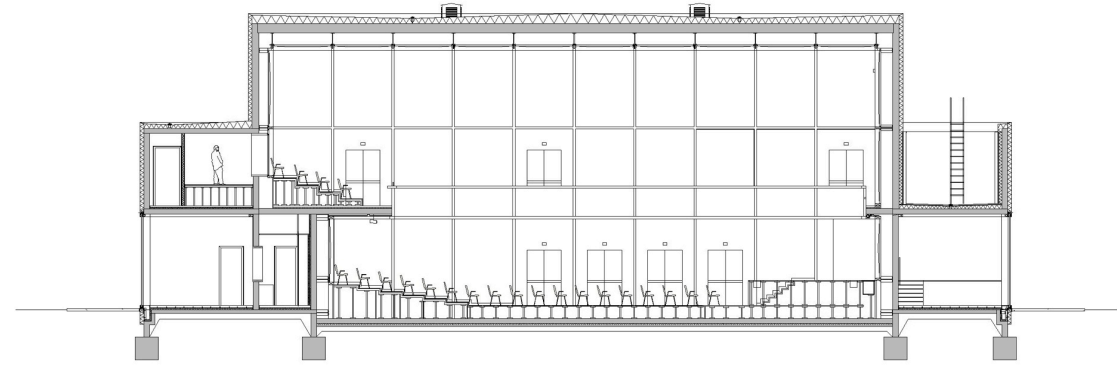
Liszt-központ, hangversenytér, Raiding, Atelier Kempe Thill, 2005
