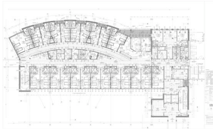
4.04. Double corridor plan, Szt Imre Hospital, Budapest (2008.) Arch.: SCHRAMMEL Z.
